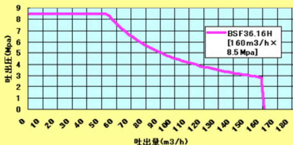
BSF36.16H/BSF28.16H ポンプ能力比較線図
